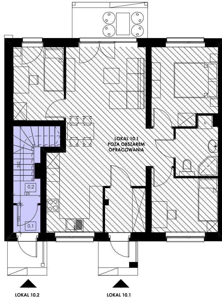
RZUT PARTERU
